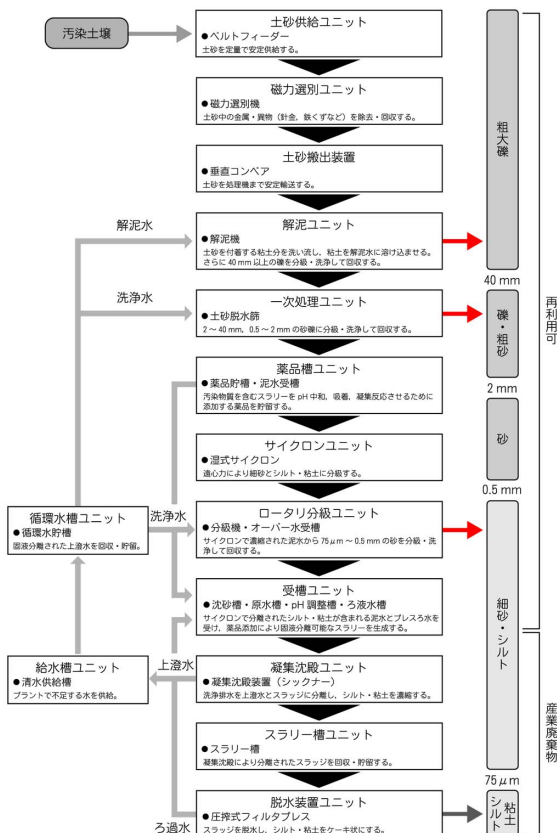
図6 土壌洗浄分級処理設備処理フロー 6)
